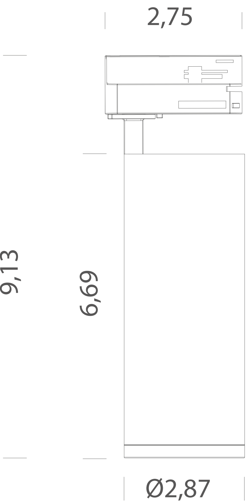
Capri TRIAC
