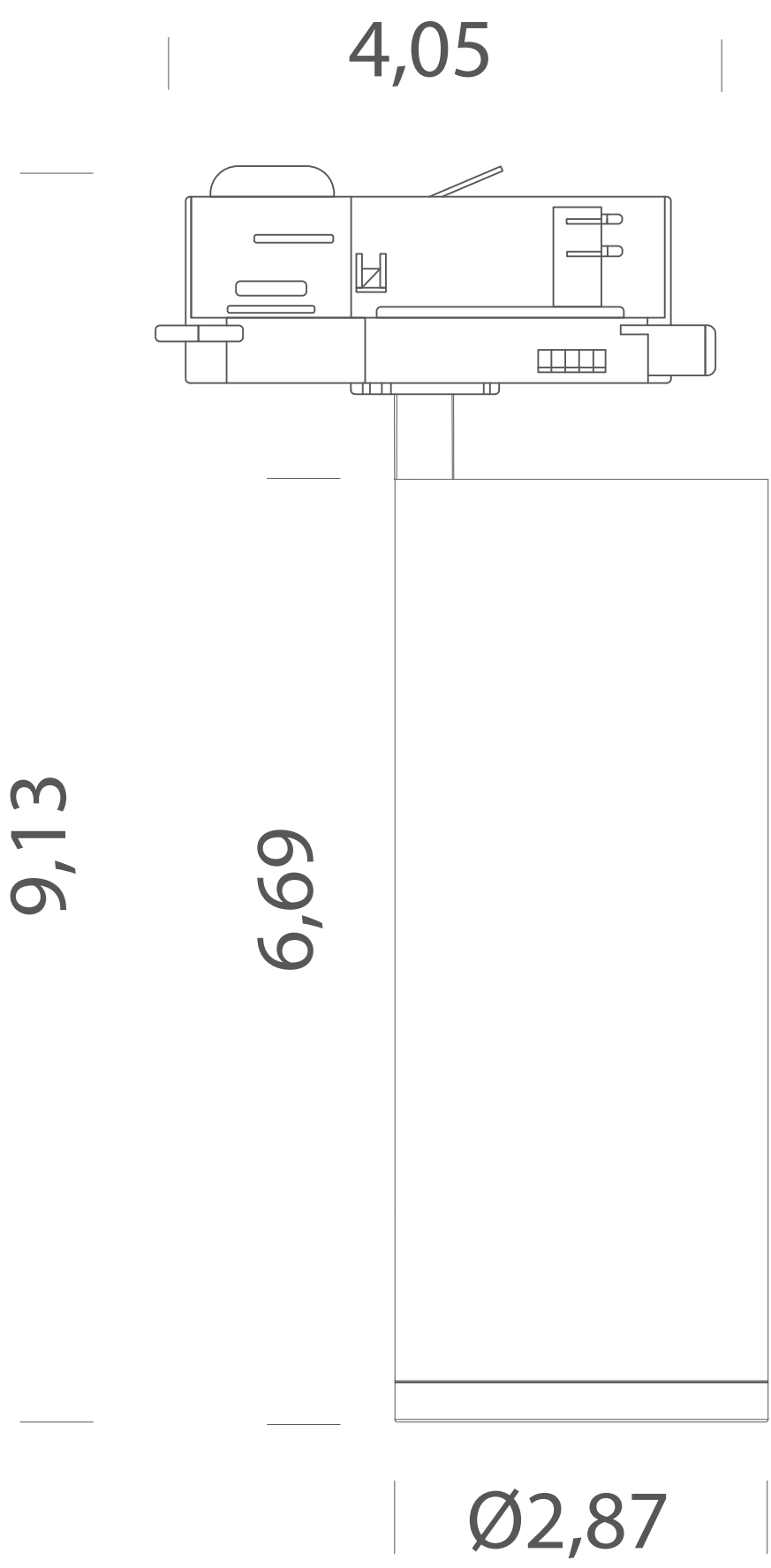
Capri DALI/1-10V
