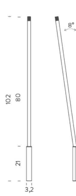
MINIFLUX LINEA WALL 8°
