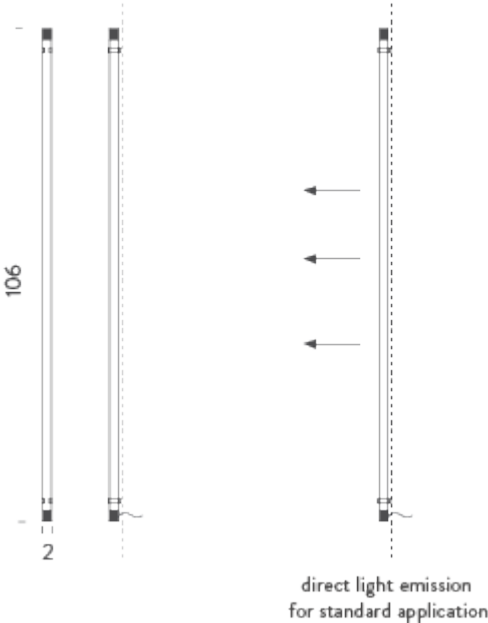
MINIFLUX LINEA WALL - C opal
