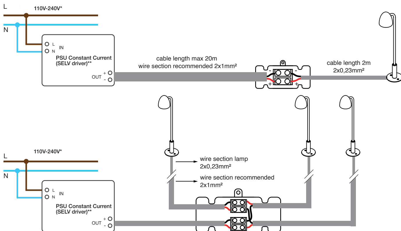
Diagramma di collegamento in serie / Series wiring diagram
